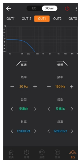
分频器
